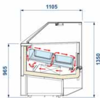
Maßzeichnung
