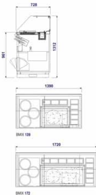
Maßzeichnung
