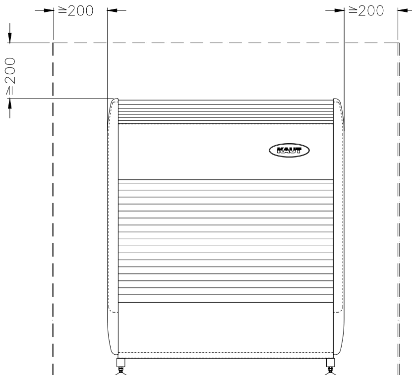
Abb.1: einzuhaltende Abstände
