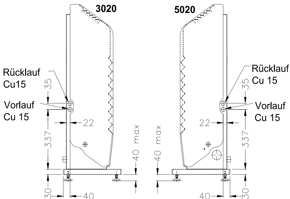
Abb. 7: Position der Heizungsanschlüsse
